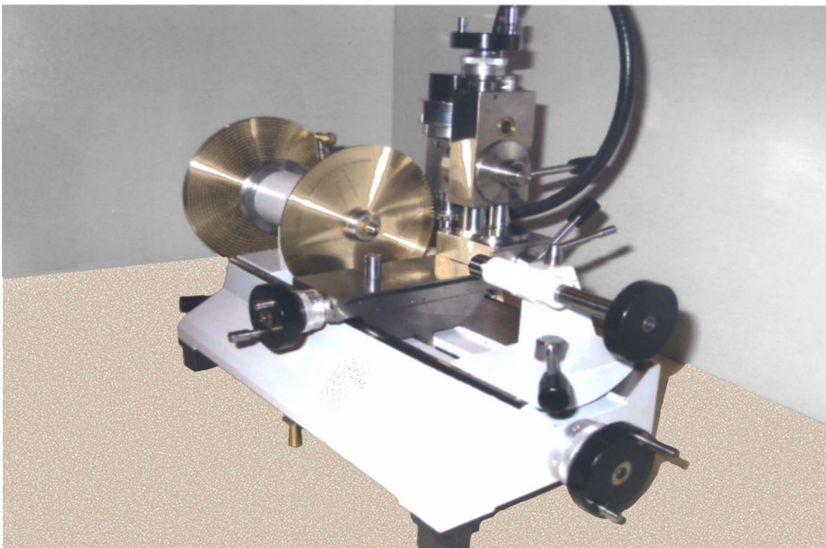
Esecuzione di una ruota dentata al massimo diametro (mm 122)
