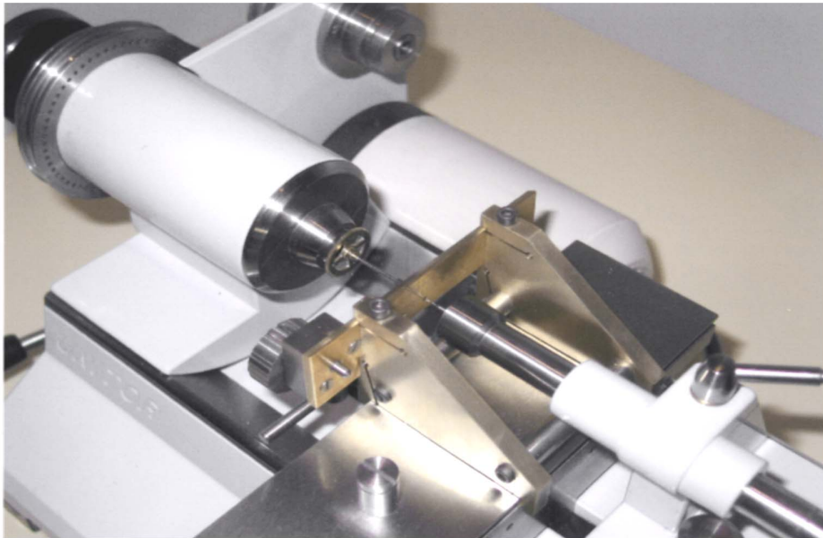
Foratura della ruota per riporto perno
