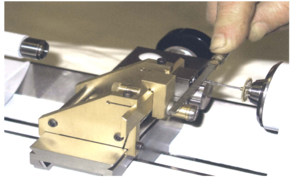
Pivottatura del perno con dispositivo
